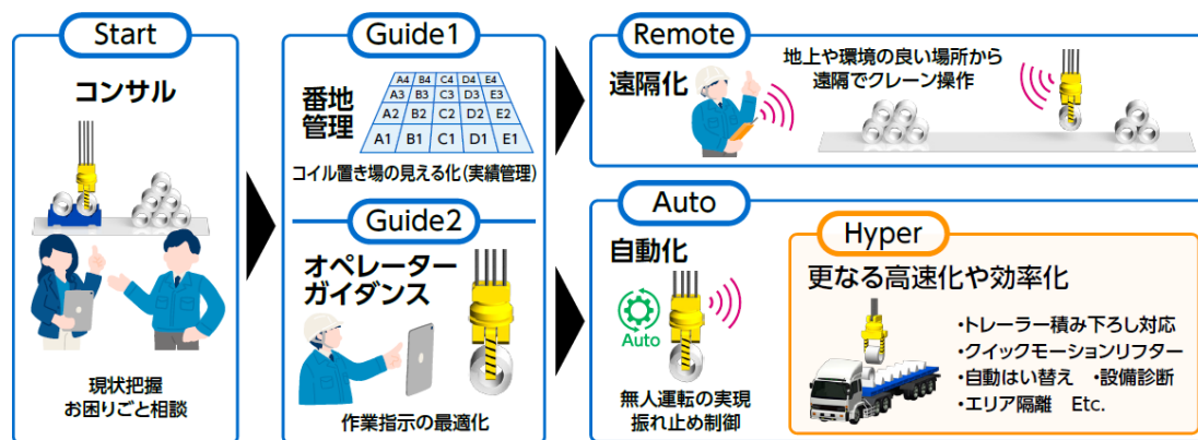
【図 1】自動クレーンシステムを中核とした倉庫ソリューション全体像
