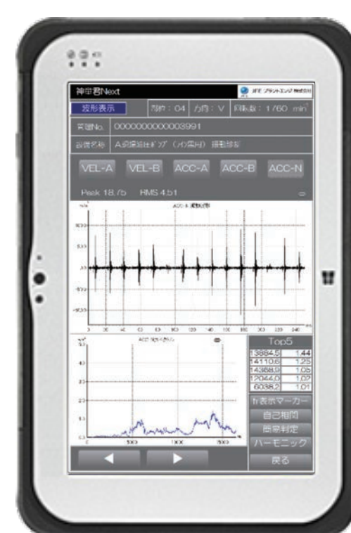
◆頑丈タブレットPC(10.1型)
