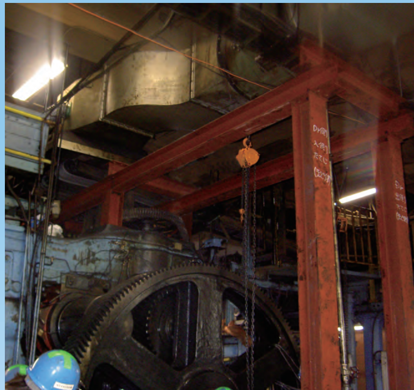
加圧ロール式ゴム成型 プレスの大ギヤ交換
