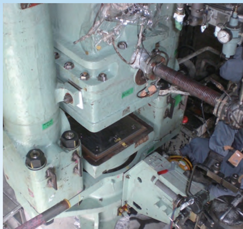
粉体成形プレスの整備移設 (能力増強含む)
